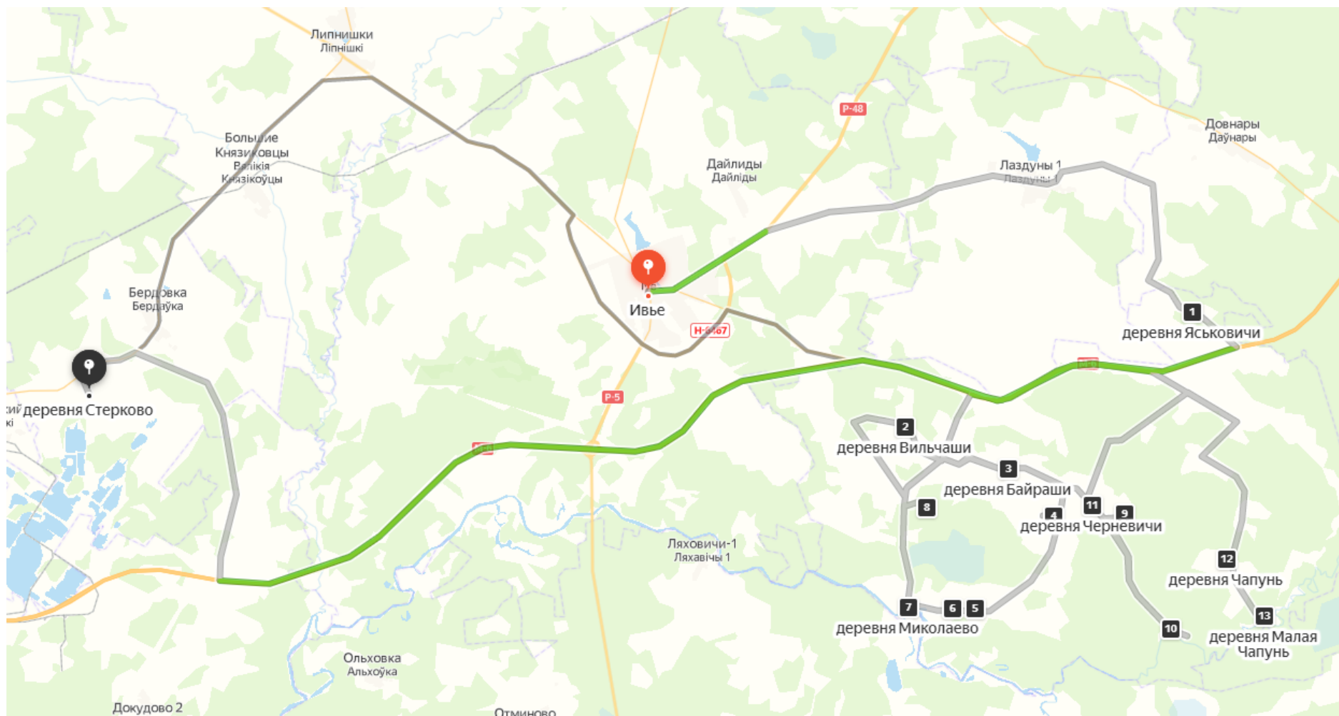
Рисунок 32 – Маршрутный график сбора и удаления ВМР машина 2 4й пн. Рейс 1
